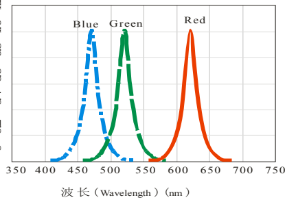
光谱分布特性曲线 Relative Spectral Distribution
